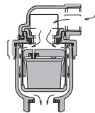
急速吸気(負圧破壊)
